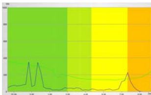
Verbrauchskurve (blau) eines Feldtesthaushaltes im Vergleich zum H0-Standardlastprofil (grün), hinterlegt mit dem Preisstufenverlauf des Tages.
